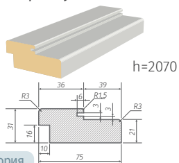
Коробочный брус прямоугольный
