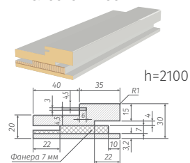
Коробочный брус (сэндвич) телескопический
